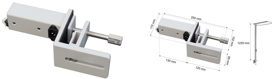
Systembild
