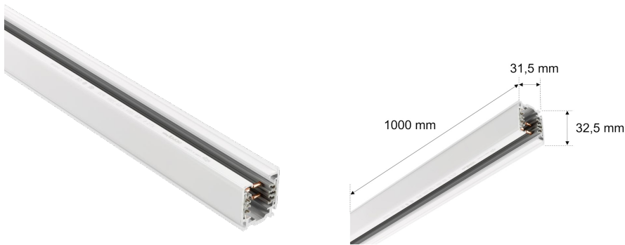
Systembild
